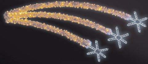
★ Art. Nr.: 162132130 ca. 100 cm x 230 cm 396 LEDs · 20,4 W · 6 kg
