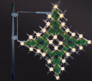
★ Art. Nr.: 8528LEDW 100 cm x 100 cm 28 Brennstellen 19,6 W · 5 kg
