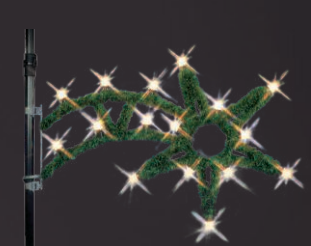
★ Art. No.: 8516LEDW 120 cm x 75 cm 16 Light bulbs 11,2 W · 4,5 kg
