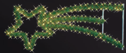
Art. No.: 94105LEDW 150 cm x 60 cm 180 LEDs · 9 W · 3,5 kg
