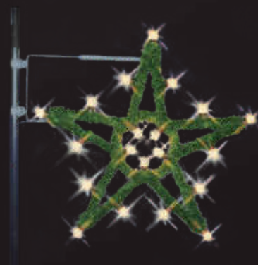
Art. No.: 8520LEDW 95 cm x 95 cm 20 light bulbs · 14 W · 4 kg
