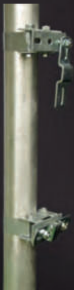
Art. Nr.: MS-2 Spannbandschelle und Klemmplatte für Mastmontage ab 6 cm, Set mit 2 Stück
